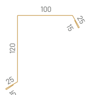
Wiatrownica boczna F02
